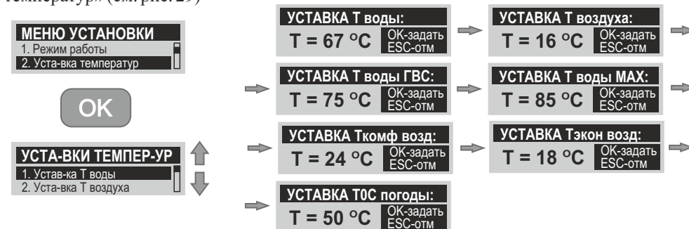
Рисунок 29. Установка температурных параметров.
