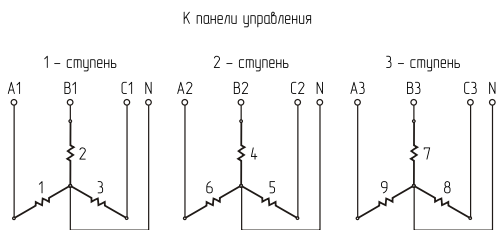
Подключение «Звезда» ZOTA «Prom» 60 - 100
