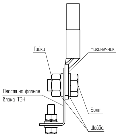
Рис.3 Присоединение проводов к выводам блок ТЭН
