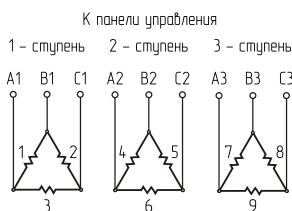
Подключение «Треугольник» ZOTA «Prom» 160 - 400
