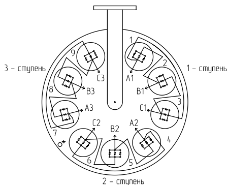
Рис.2 Расположение выводов и схема подключения котла.
